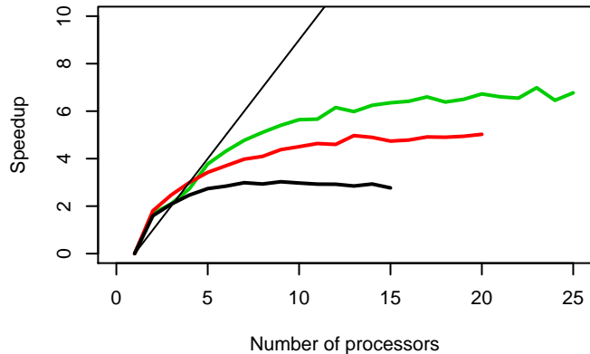
BGCorrection (RMA)
