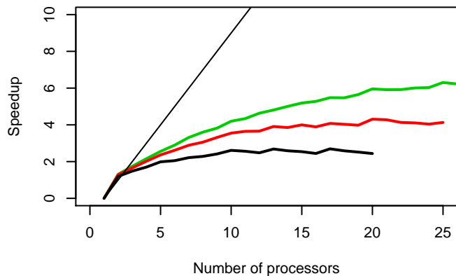
BGCorrection (RMA)
