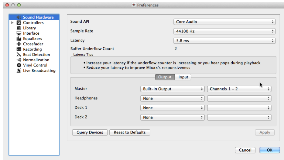
Figure1: Utilizare Mixxx cu placa de sunet inclusă
