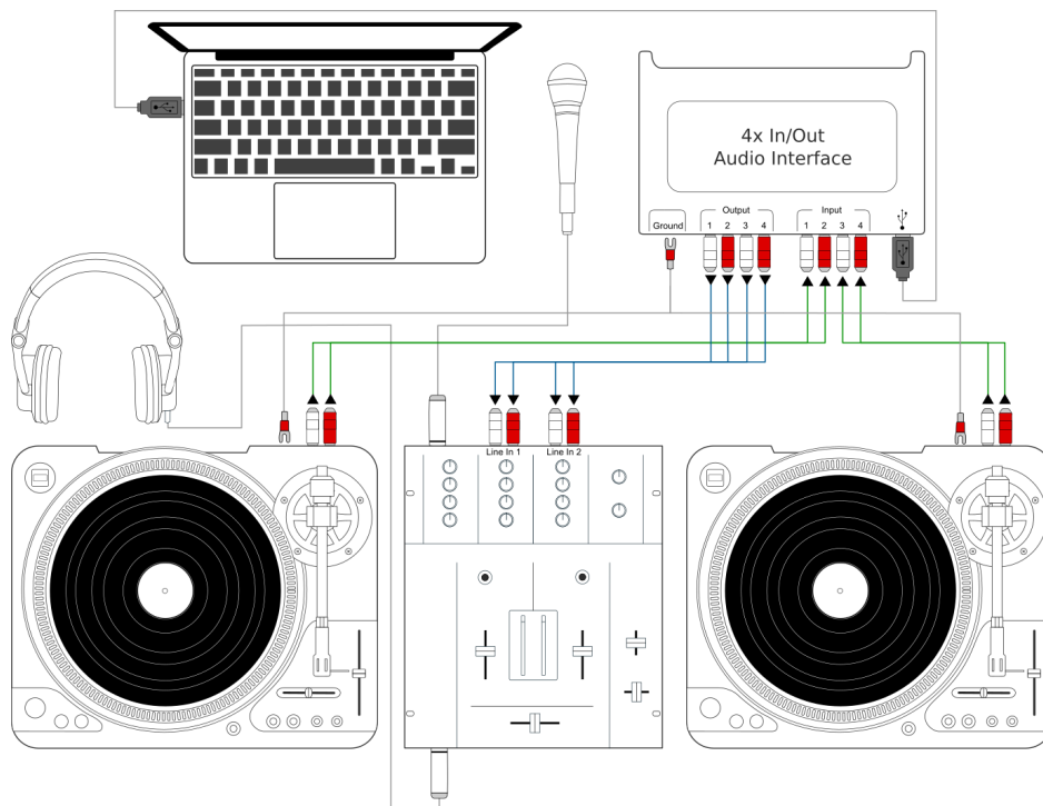
Figure5: Utilizarea Mixxx împreună cu platane și mixere externe
