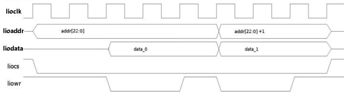
图13- 2 LocalI/O 写时序
