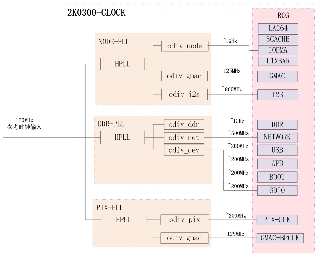
图2- 1 时钟结构
