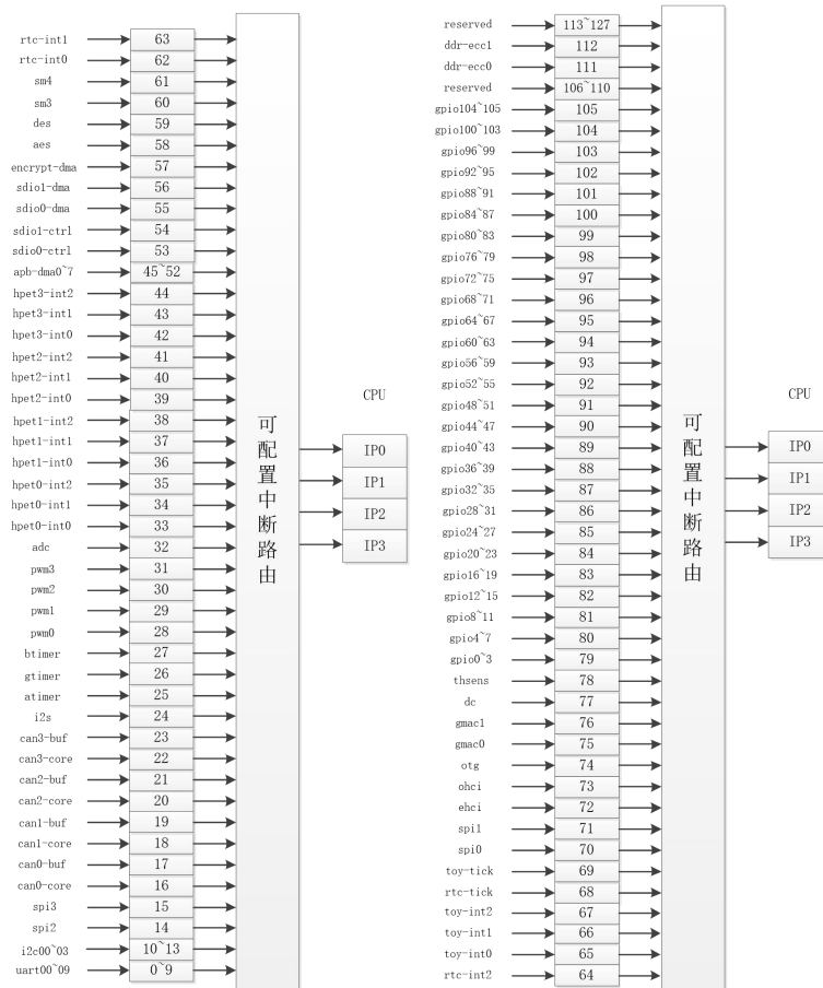
图3- 3 龙芯 2K0300 扩展 IO 中断路由示意图
