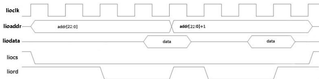
图13- 1 LocalIO 读时序
