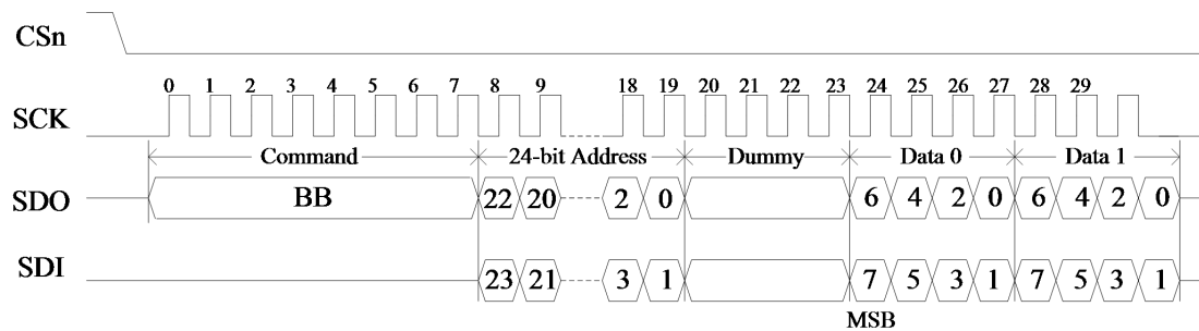
图9- 5 SPI Flash 双向 I/O 读时序
