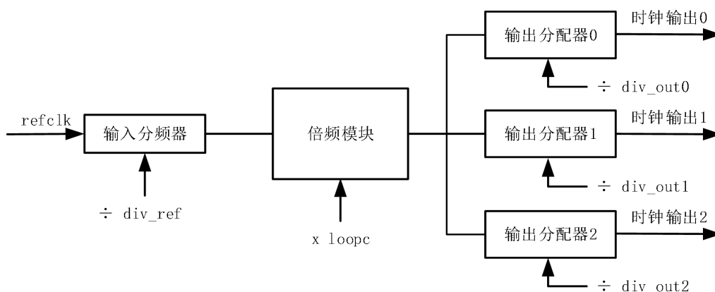
图3- 1 展频 PLL 概念性结构
