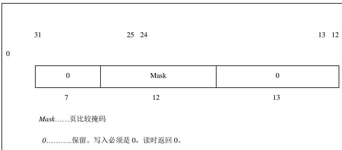
图 5-7 PageMask 寄存器
