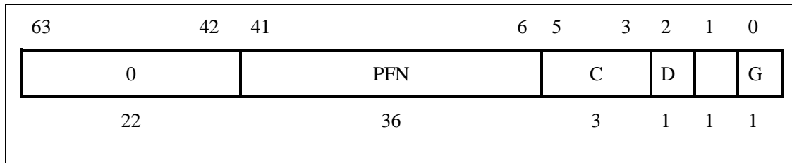
图 3-3 EntryLo0 和 EntryLo1 寄存器
