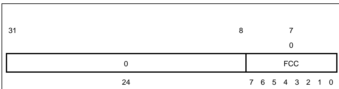
图 7-5 FCCR 寄存器
