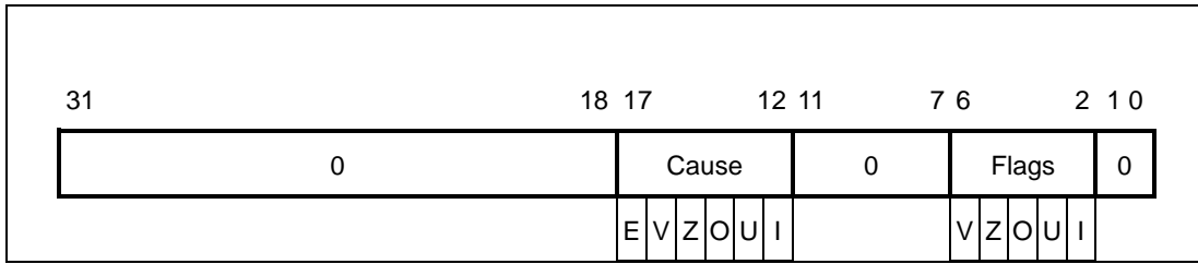
图 7-6 FEXR 寄存器
