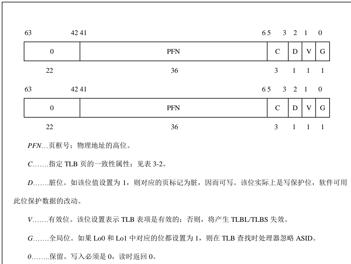
图 5-9 EntryLo0 和 EntryLo1 寄存器
