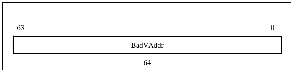
图 3-10 BadVAddr 寄存器
