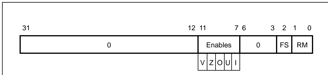
图 7-7 FENR 寄存器
