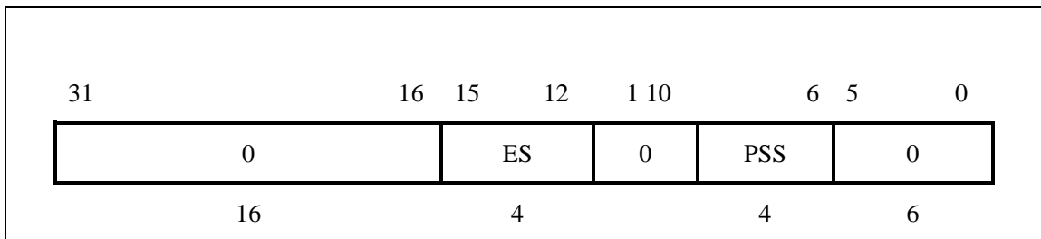
图 3-16 SRSCtl 寄存器
