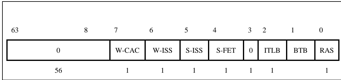
图 3-27 Diagnostic 寄存器
