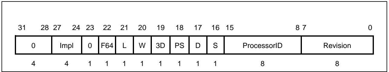
图 7-3 FIR 寄存器
