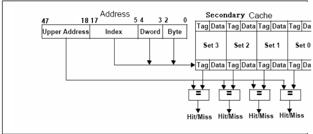
图 4-5 二级 Cache 访问
