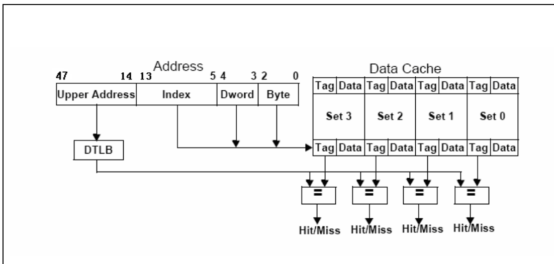
图 4-4 数据 Cache 访问
