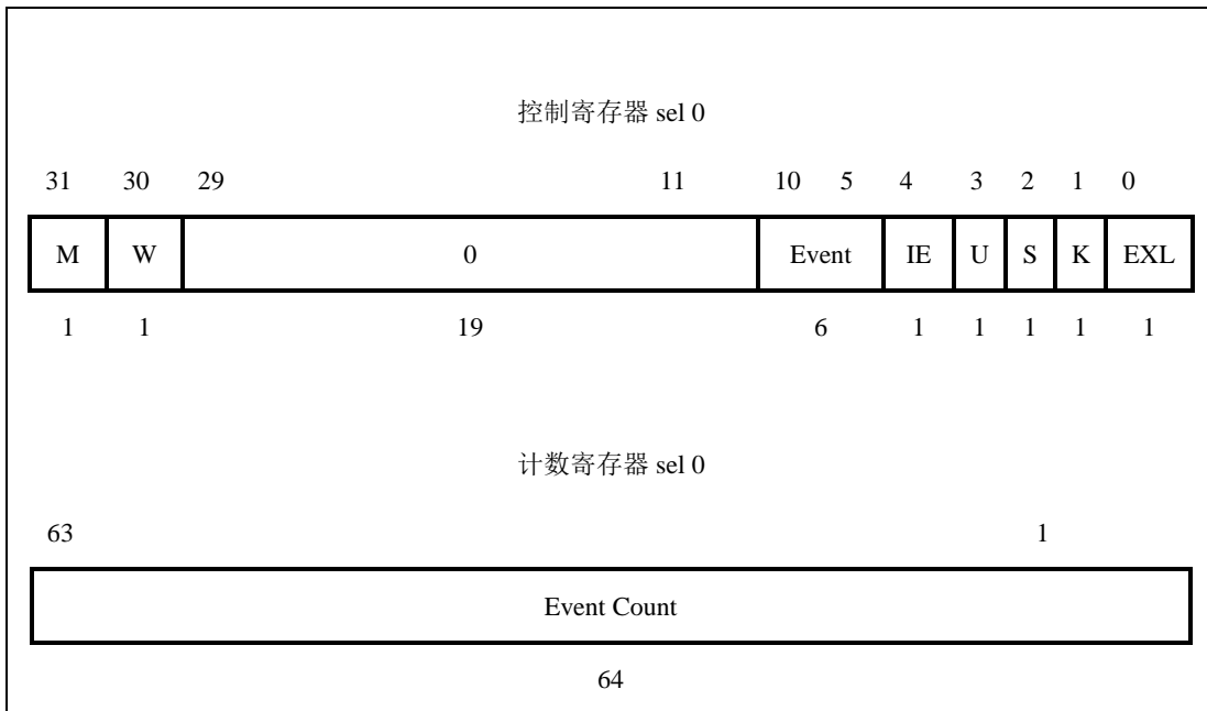
图 3-30 性能计数器寄存器
