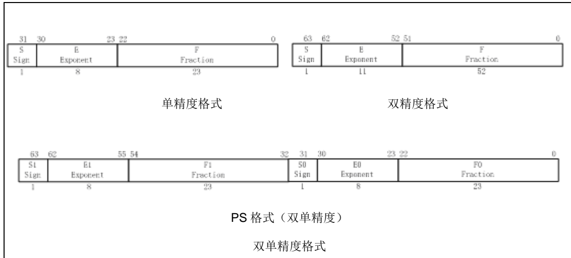
图 7-8 浮点格式
