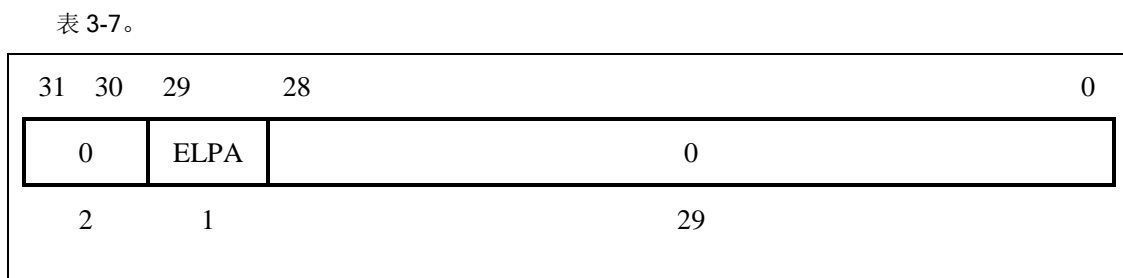
图 3-6 PageGrain 寄存器
