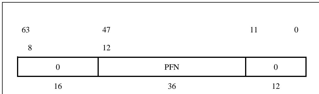
图 3-25 LLAddr 寄存器
