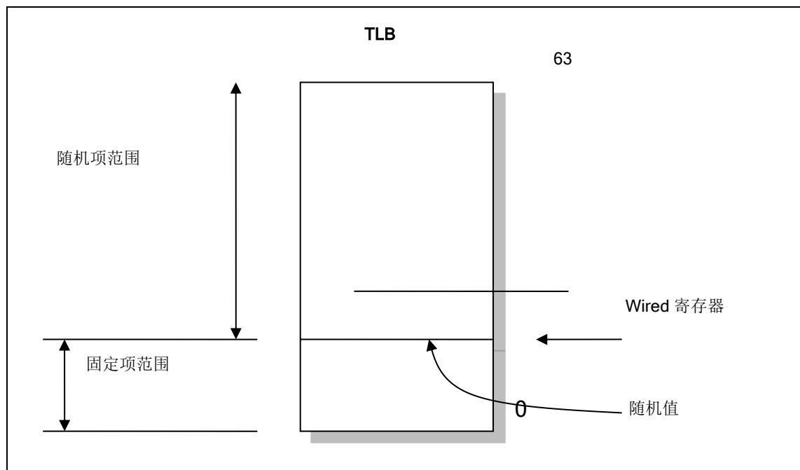
图 3-7 Wired 寄存器界限
