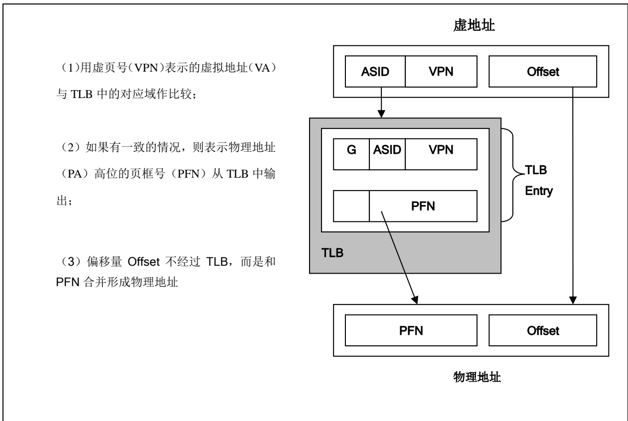
图 5-1 虚实地址转换概览
