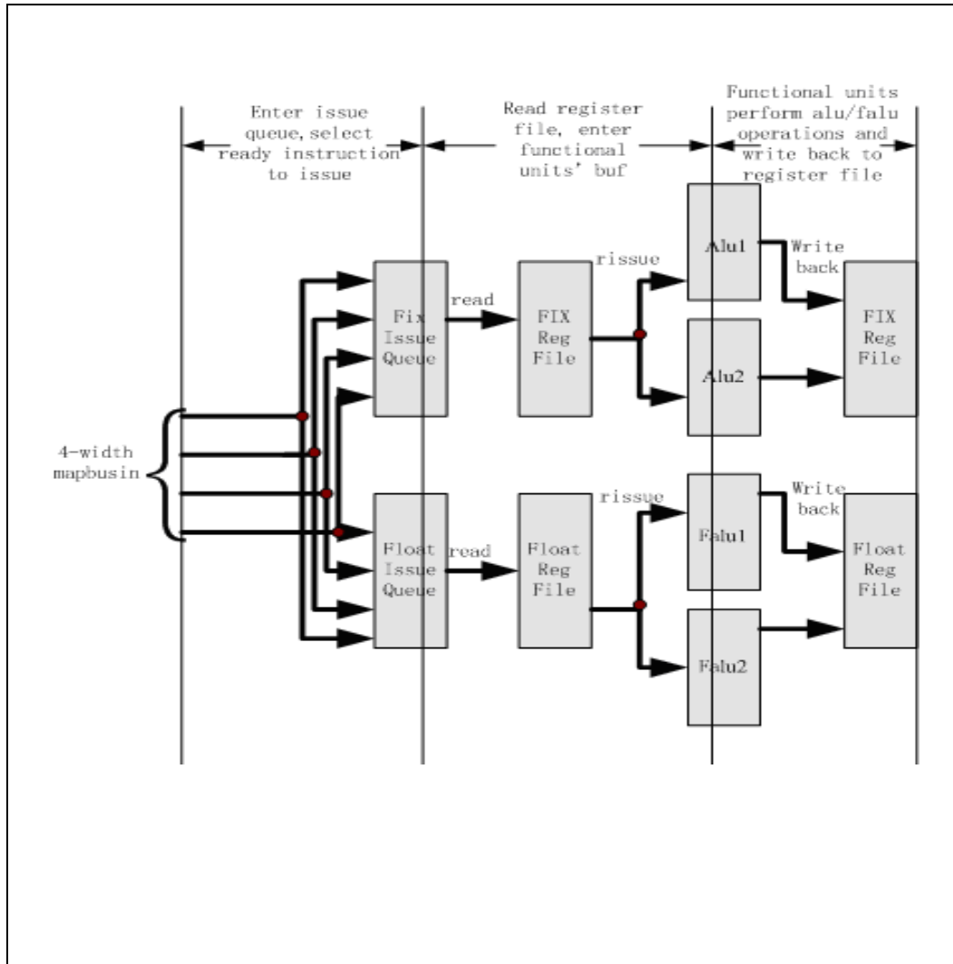
图 7-1 龙芯 3A 体系结构中功能单元的组织构成
