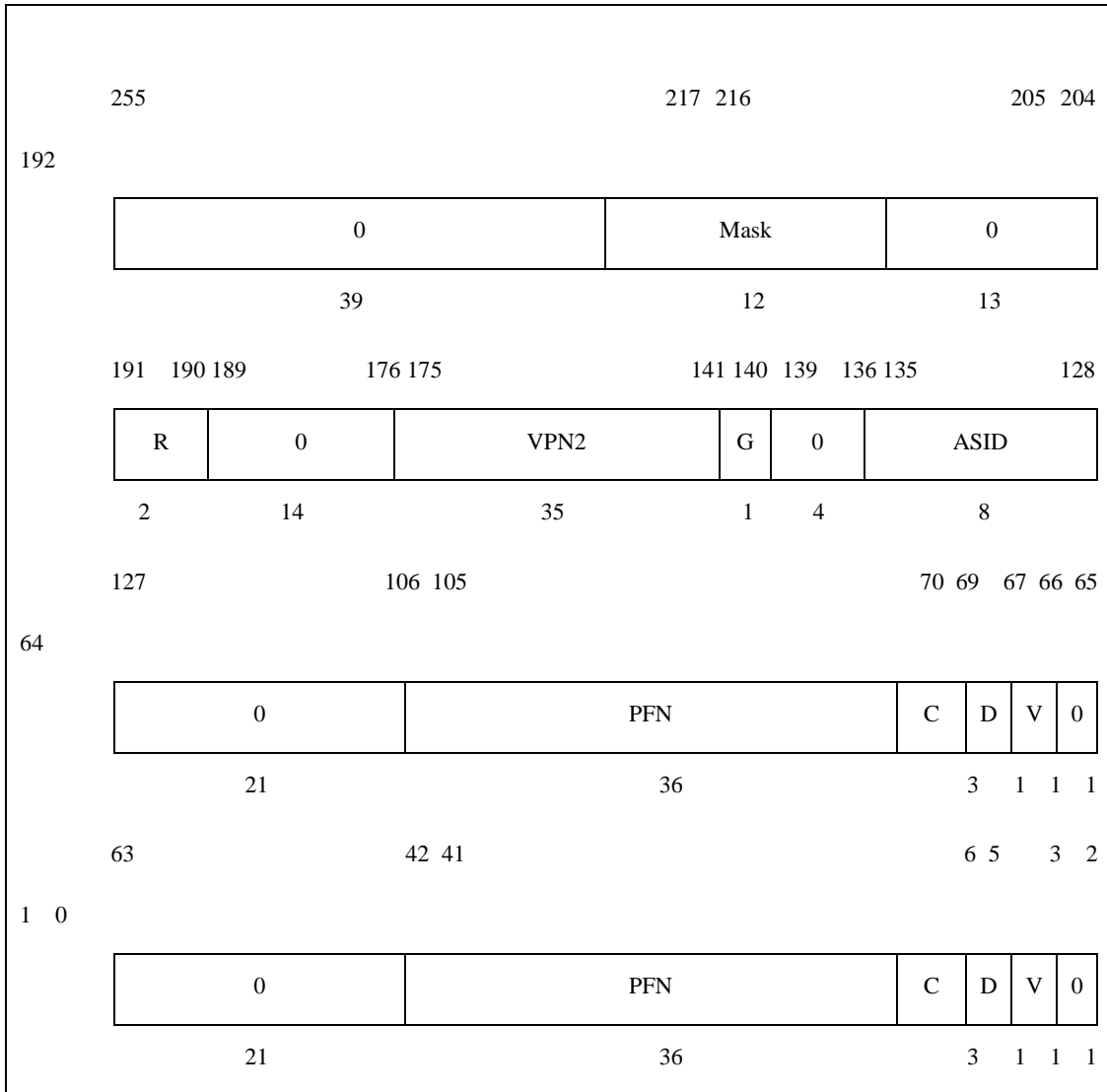
图 5-6 TLB 表项
