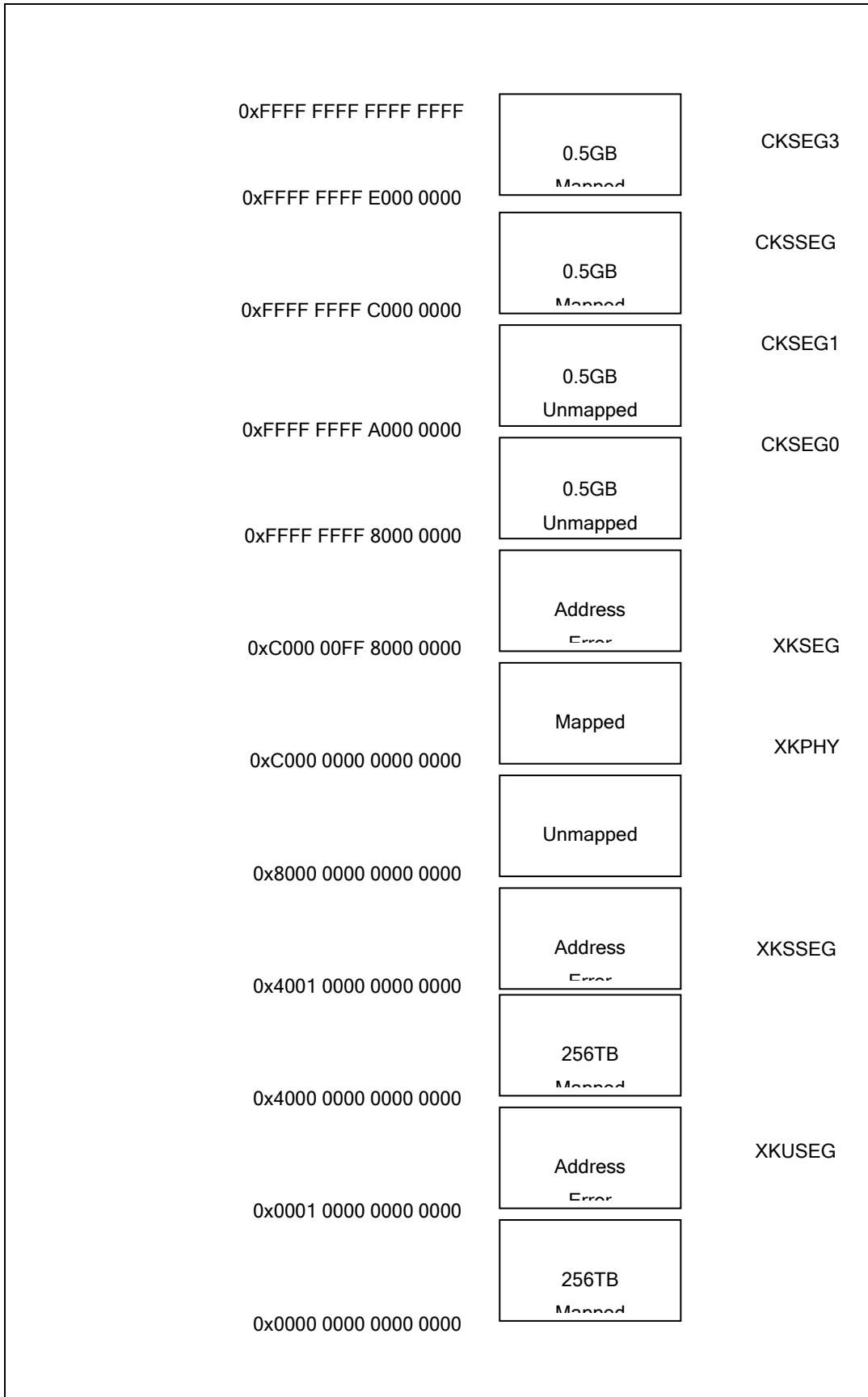
图 5-5 内核模式下的用户、管理、内核地址空间概况
