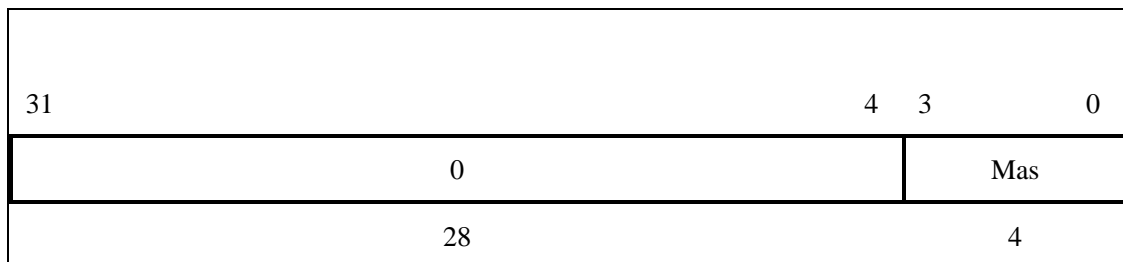
图 3-9 HWREna 寄存器
