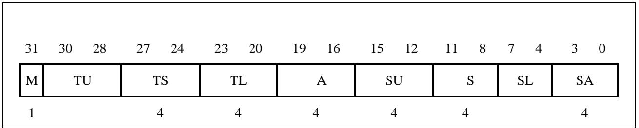
图 3-23 Config2 寄存器
