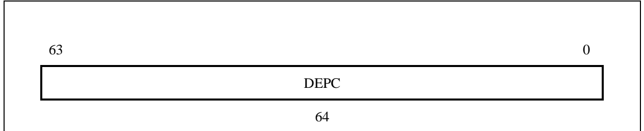
图 3-29 DEPC 寄存器
