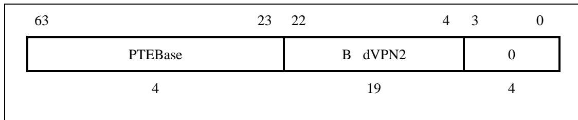
图 3-4 Context 寄存器
