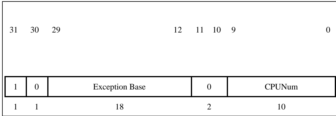
图 3-20 Ebase 寄存器
