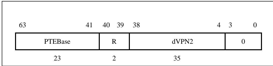
图 3-26 XContext 寄存器
