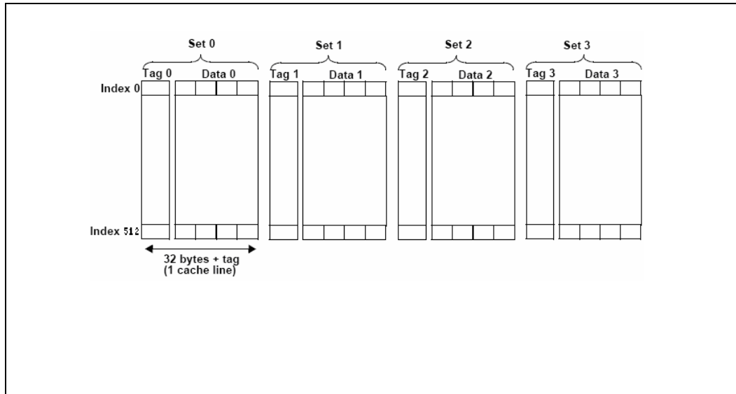
图 4-1 指令 Cache 的组织
