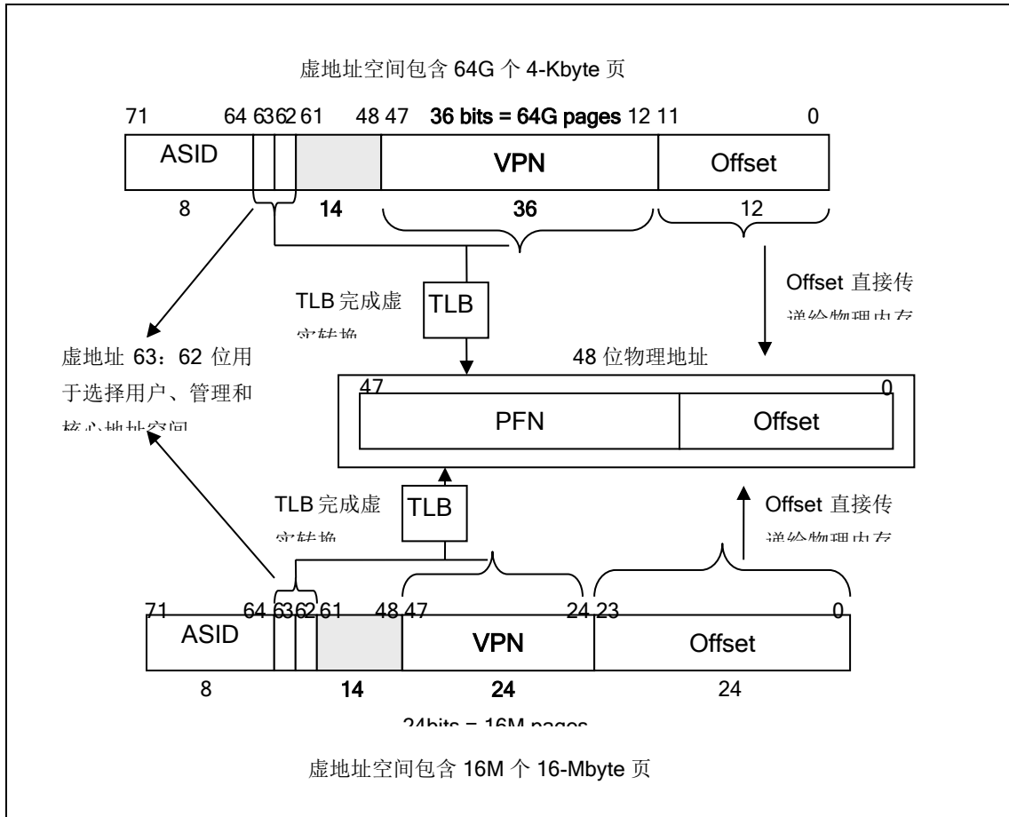
图 5-2 64 位模式虚拟地址转换
