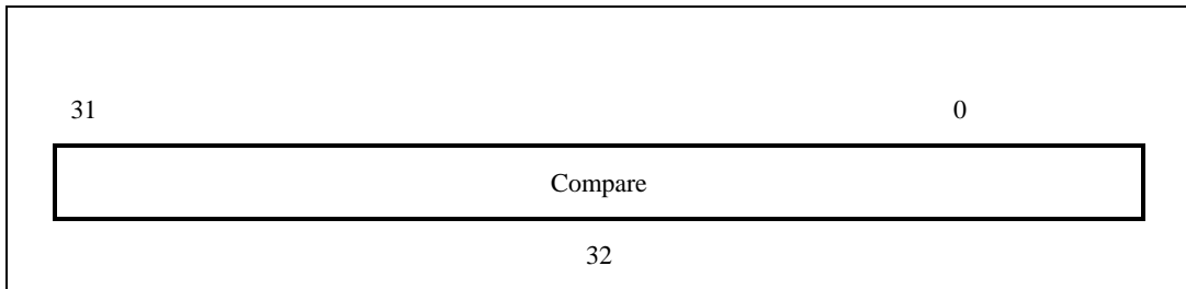
图 3-12 Compare 寄存器
