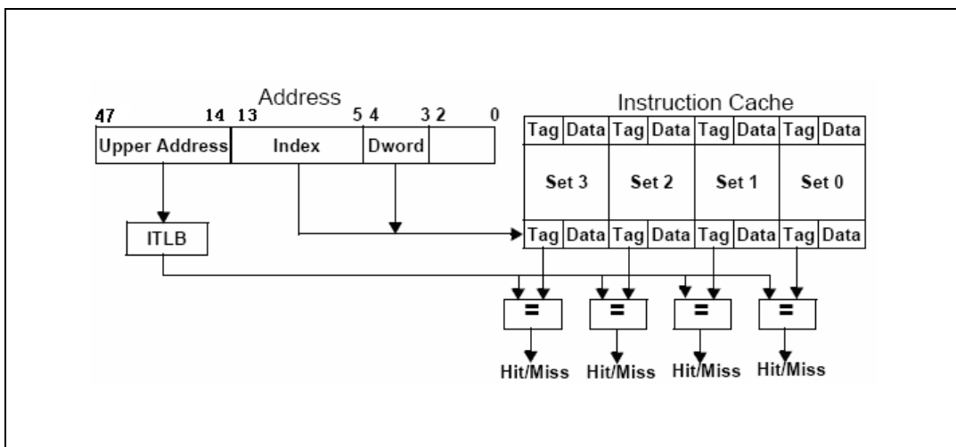
图 4-2 指令 Cache 访问
