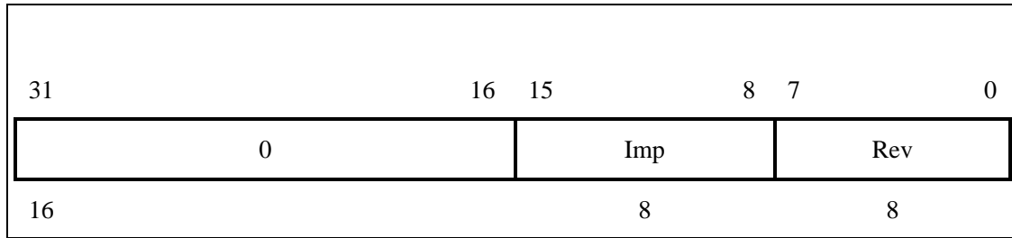
图 3-19 Processor Revision Identifier 寄存器
