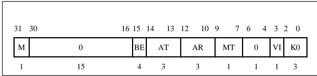
图 3-21 Config 寄存器
