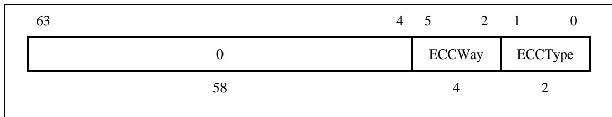
图 3-32 CacheErr 寄存器
