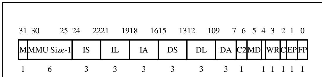
图 3-22 Config1 寄存器
