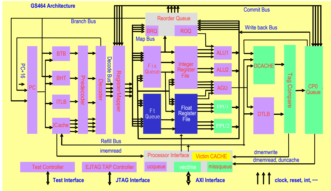
图 1-1 GS464 处理器的基本结构
