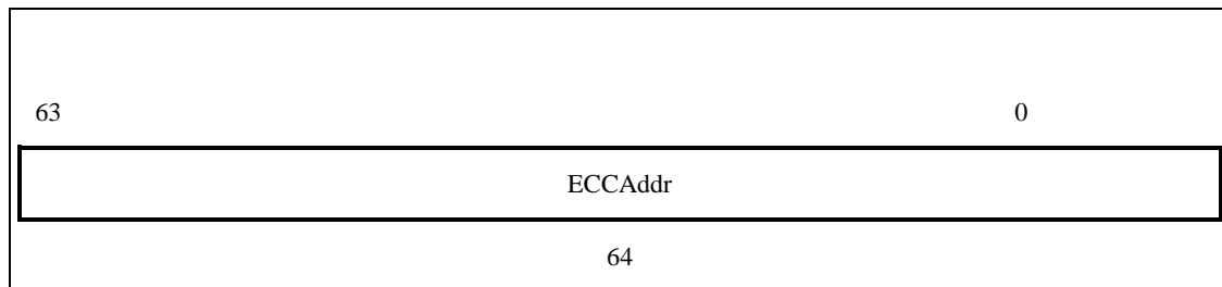
图 3-33 CacheErr1 寄存器
