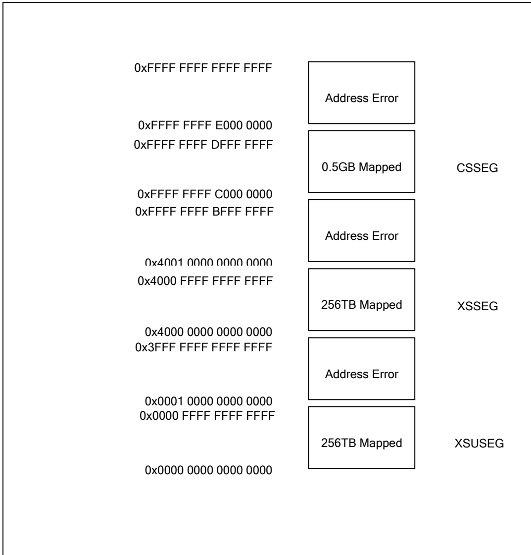
图 5-4 管理模式下用户空间和管理空间
