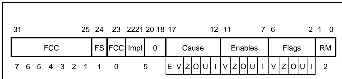
图 7-4 FCSR 寄存器
