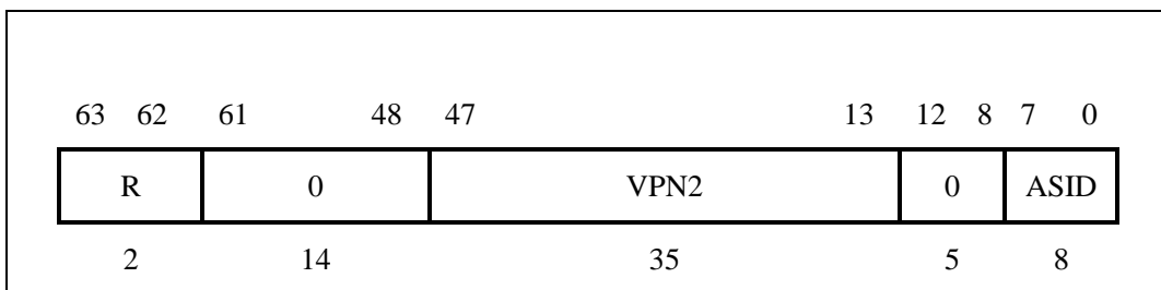
图 3-13 EntryHi 寄存器
