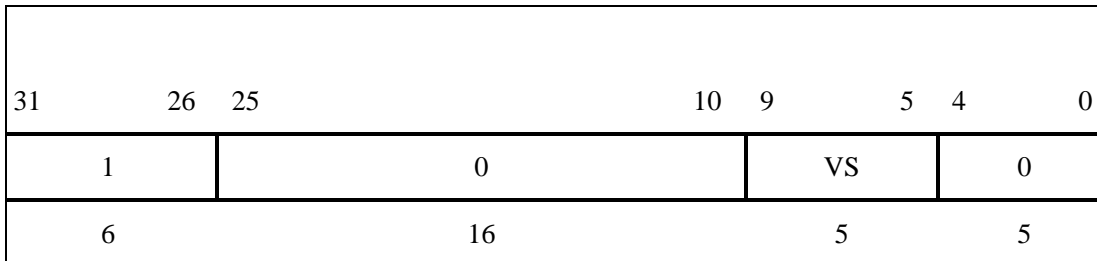
图 3-15 IntCtl 寄存器
