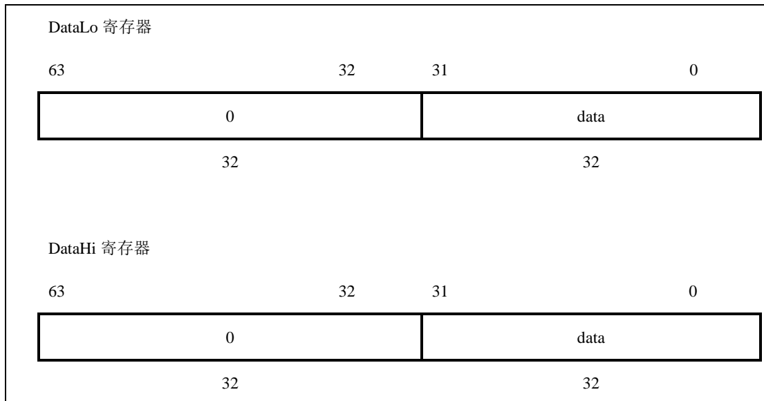
图 3-36 DataLo 和 DataHi 寄存器
