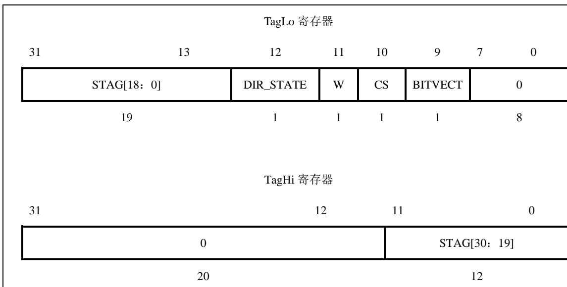
图 3-35 TagLo 和 TagHi 寄存器 (SCache)
