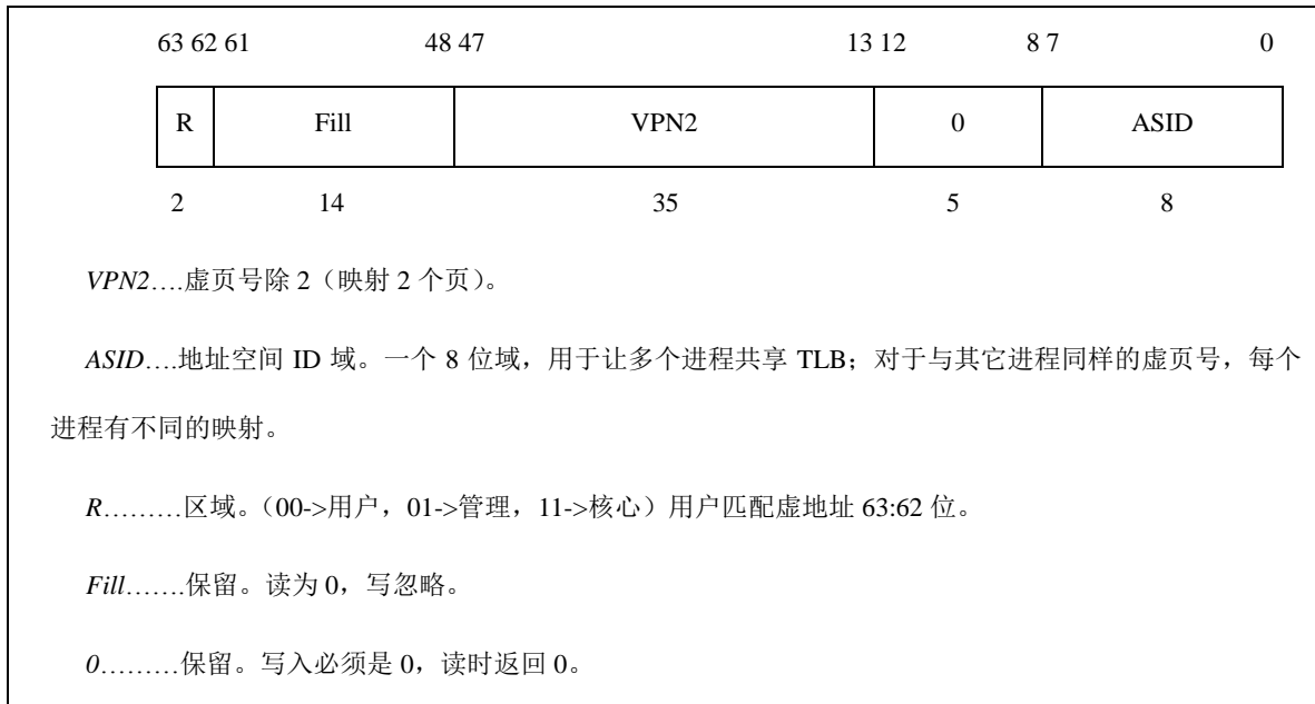
图 5-8 EntryHi 寄存器
