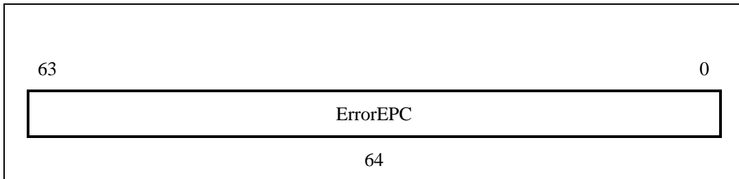
图 3-37 ErrorEPC 寄存器
