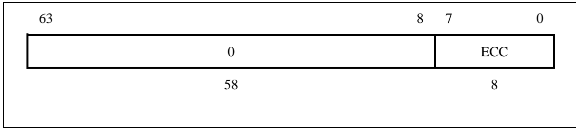
图 3-31 ECC 寄存器
