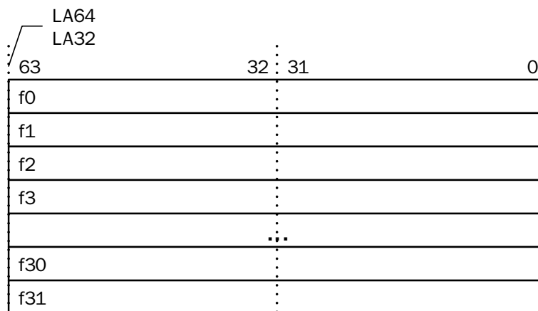
图 3- 1 浮点寄存器
