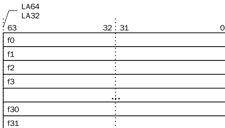
图 3- 1 浮点寄存器
