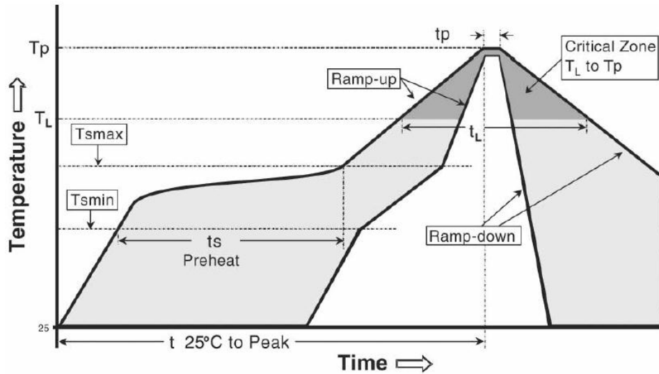
图 25.1 焊接回流曲线
