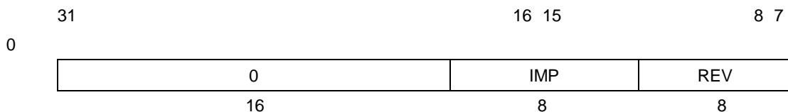
图 4-19 Processor Revision Identifier 寄存器
