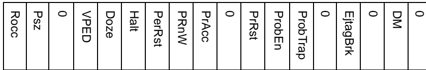
图 4-49 ECR 格式
